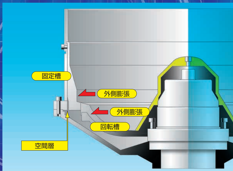
クリアランスコントロール機構
