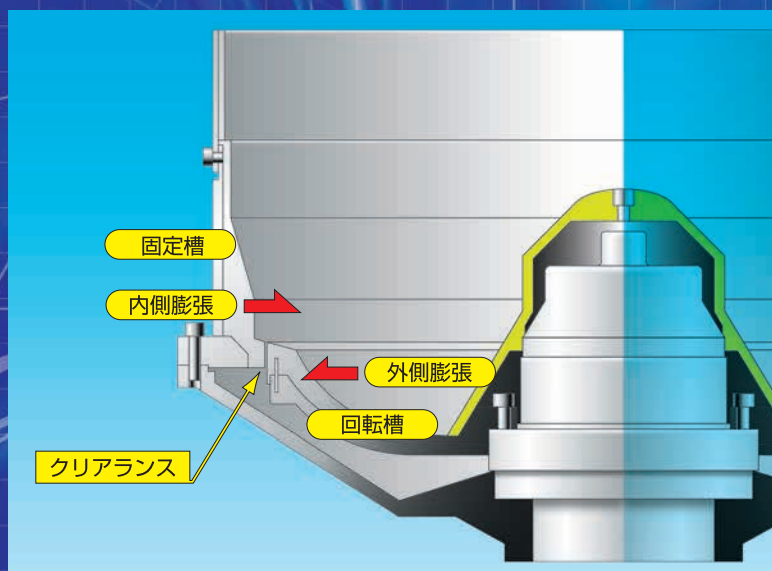
従来型のバレル槽
