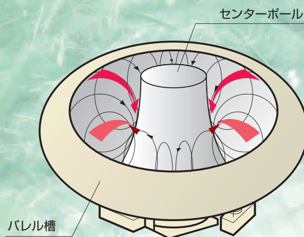
サークル型振動バレル
