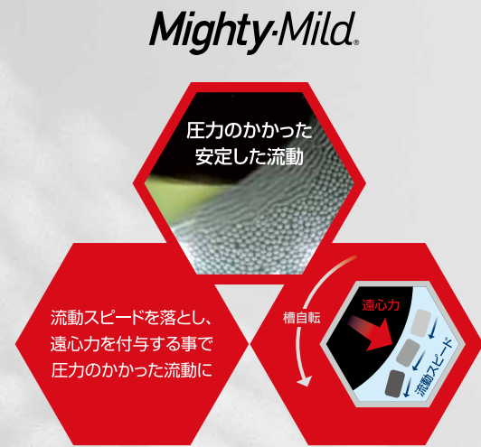
遠心バレル研磨機
