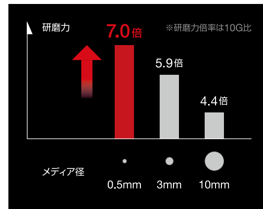
重圧化(10G→40G)による研磨力の影響
