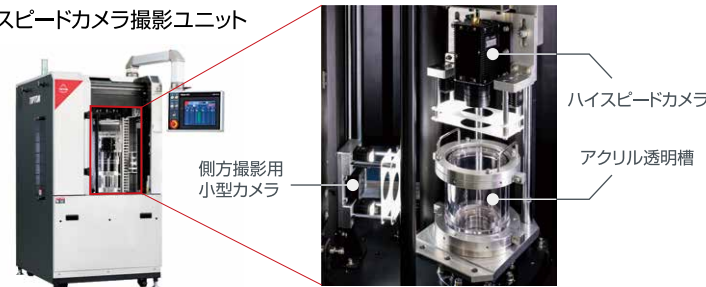
ハイスピードカメラ撮影ユニット
