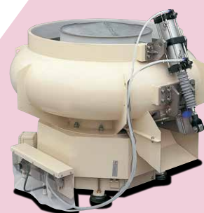
粉掛け専用機 振動式パウダーコーティングマシン Coaterow CCM キャンディコーティング
