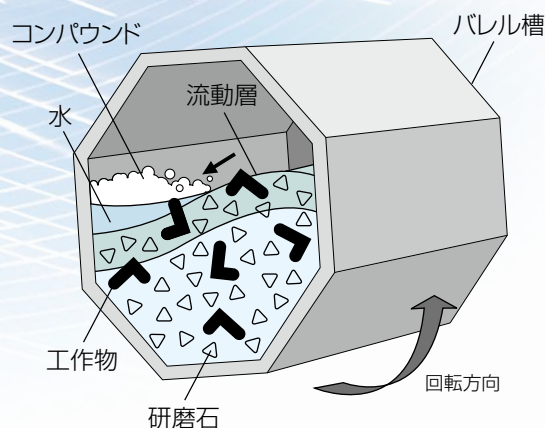
■回転バレルの流動形態
